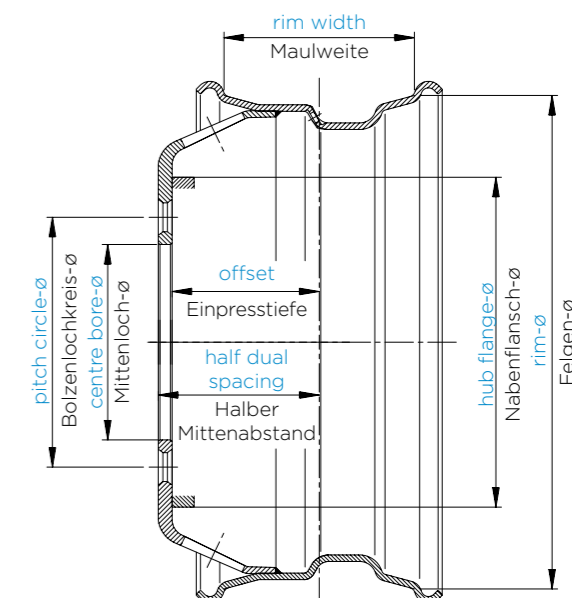
SCHEIBENRAD FÜR ZWILLINGSMONTAGE MIT 15° STEILSCHULTERFELGE FÜR SCHLAUCHLOSE BEREIFUNG
