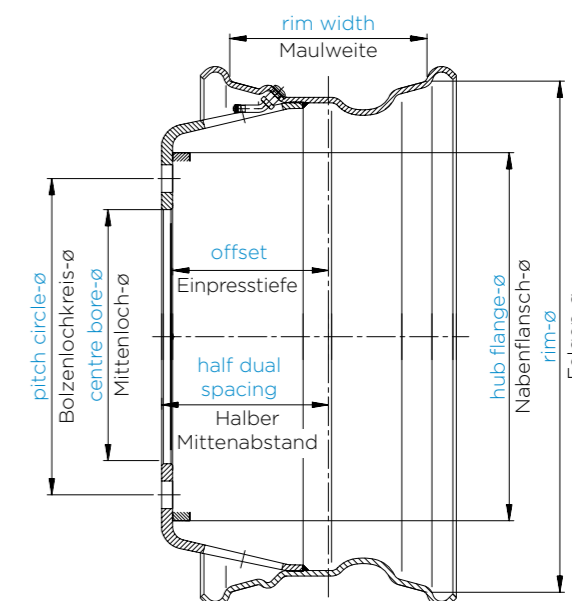
alive SCHEIBENRAD FÜR ZWILLINGSMONTAGE MIT 15° STEILSCHULTERFELGE FÜR SCHLAUCHLOSE BEREIFUNG
